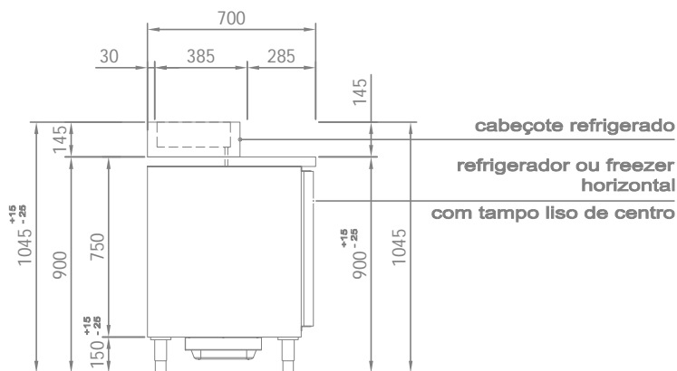
VISTA LATERAL
