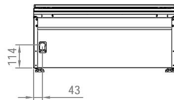
CONEXÃO DE GÁS 1/2" BSP VISTA TRASEIRA
