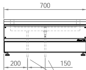
TUBULAÇÃO DA REFRIGERAÇÃO
