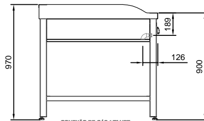
CONEXÃO DE GÁS 1/2" NPT VISTA LATERAL
